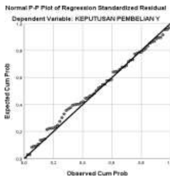
Gambar 1. 2 Tes Normalitas
