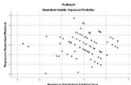
Gambar 1. 3 Pengujian Heteroskedastisitas
