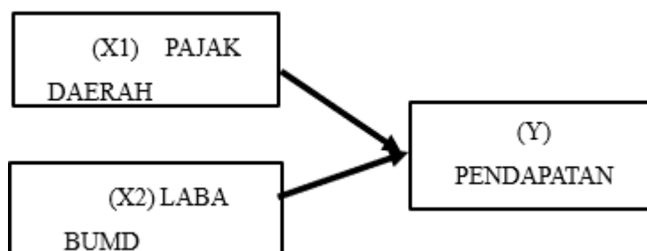
Gambar 2. 1 Kerangka Pemikiran
