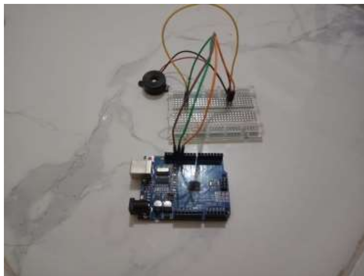
Gambar 4.8 Susunan hardware
