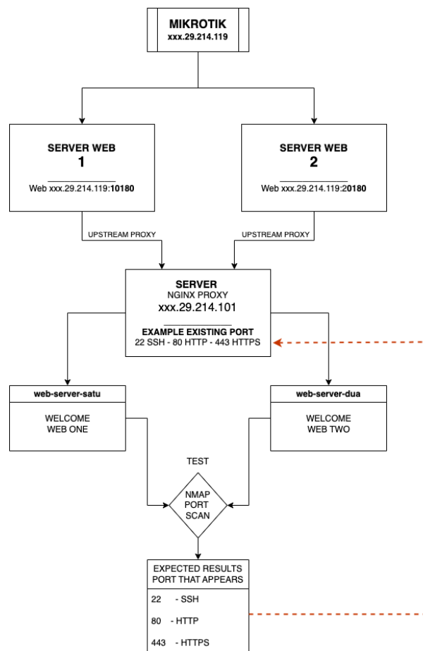
Gambar 2. Alur Penelitian: Optimasi IPv4 dan Perlindungan Terhadap NMAP Port Scan
