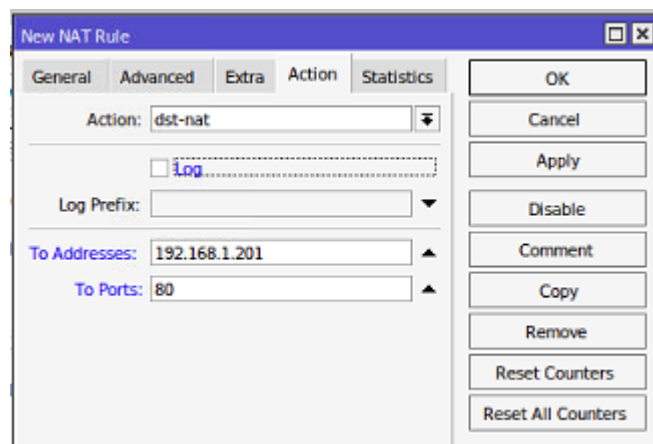
Gambar 3. Konfigurasi MikroTik IP NAT untuk server satu 192.168.1.201 dan port 80
